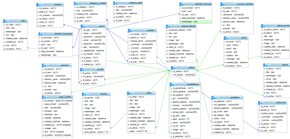
Gambar 3.5. ERD website Dinkes Prov.Sumatera Barat
