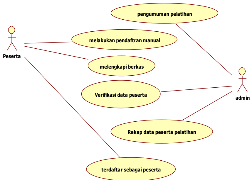
Gambar 3.2. Usecase Diagram pendaftaran
