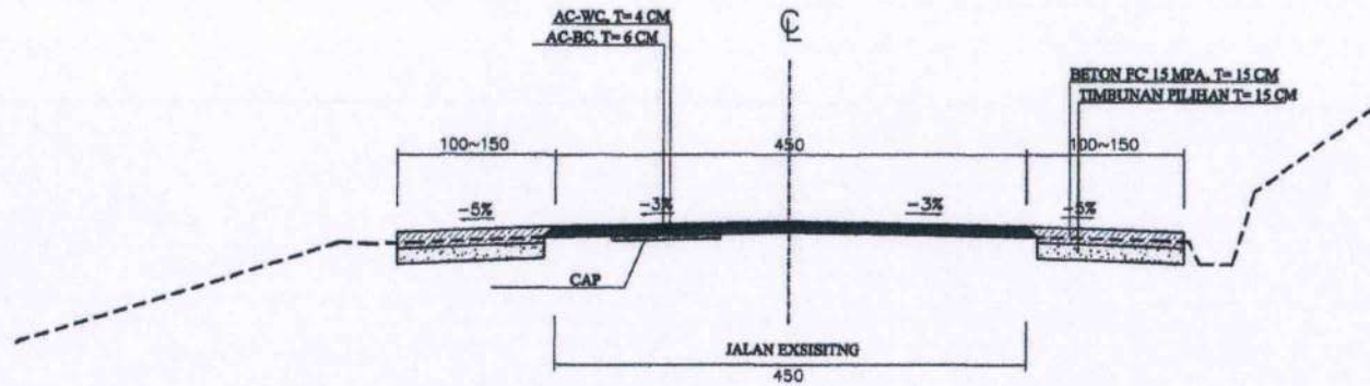
TYPICAL JALAN (STA 154+650 S/D 157+650) GRID \geq 5\%
