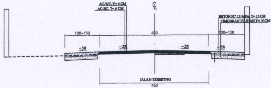
TYPICAL JALAN (STA 155+580 S/D 156+100)
