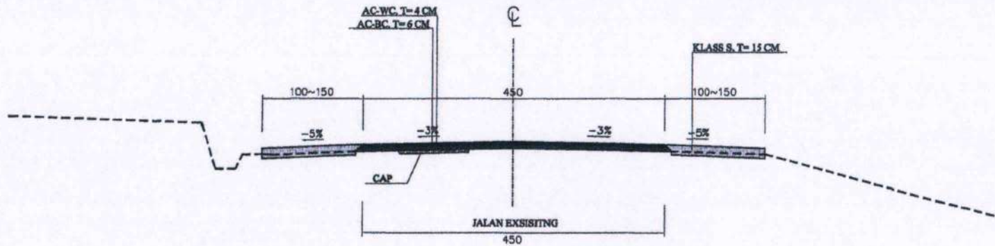
TYPICAL JALAN (STA 154+650 S/D 157+650) GRID \leq 5\%
