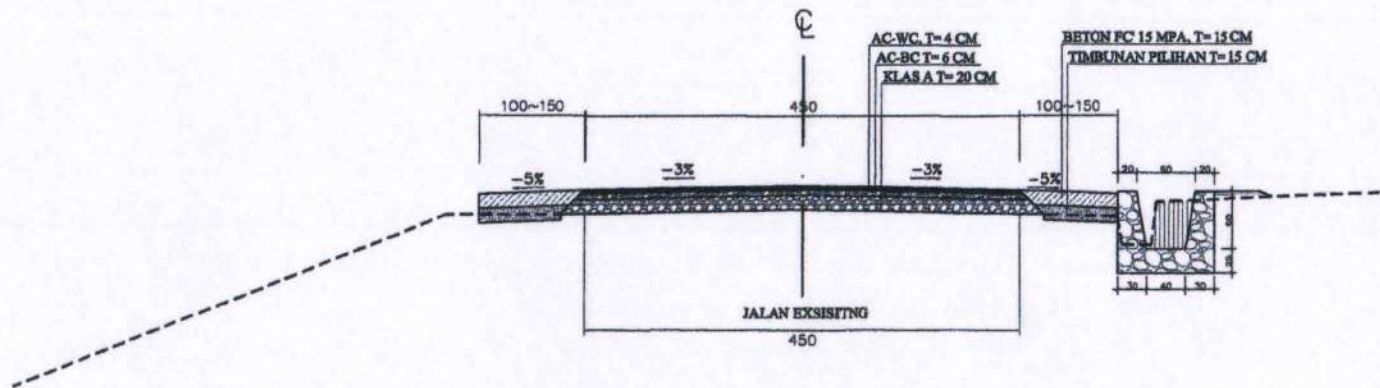
TYPICAL JALAN (STA 157+480 S/D 157+650)
