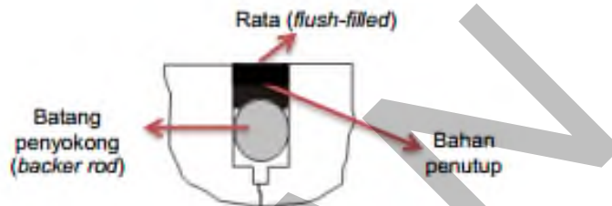
Gambar 4.12.6.1) Konfigurasi Bahan Penutup Sambungan
