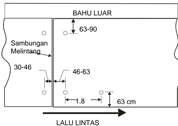
a) Rekomendasi untuk Rongga di Bawah Pelat Depan
