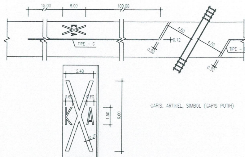
TANDA PADA PERSIMPANGAN JALAN REL KERETA API
