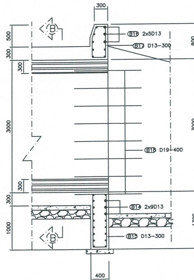
POTONGAN A - A SKALA 1:50
