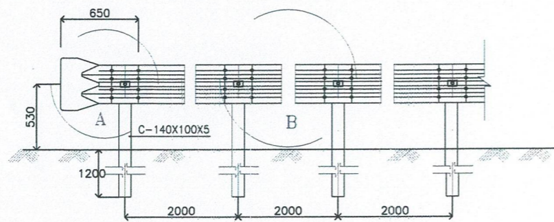
ELEVASI DEPAN
