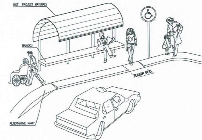
STANDAR FASILITAS PADA HALTE TANPA SKALA
