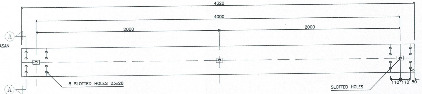
DETAIL-B
