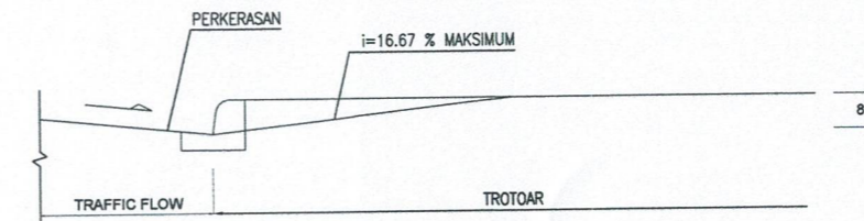
POTONGAN A-A TANPA SKALA
