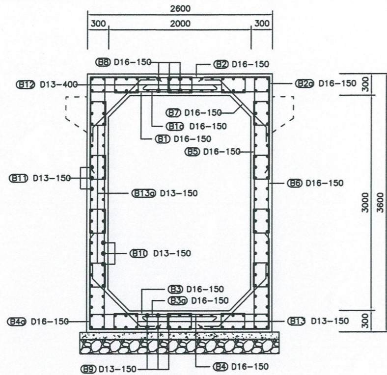
POTONGAN B - B SKALA 1:50
