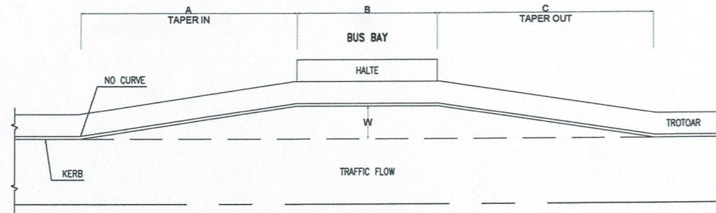
PERKERASAN KAKU TANPA SKALA
