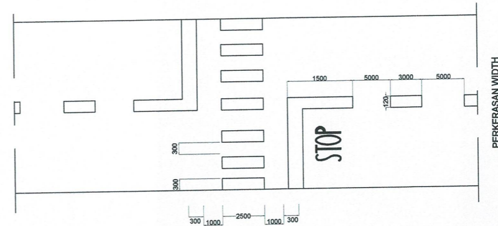
PEMBERHENTIAN DAN PENYEBERANGAN GARIS JALAN RM-5
