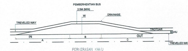
PERKERASAN KAKU
