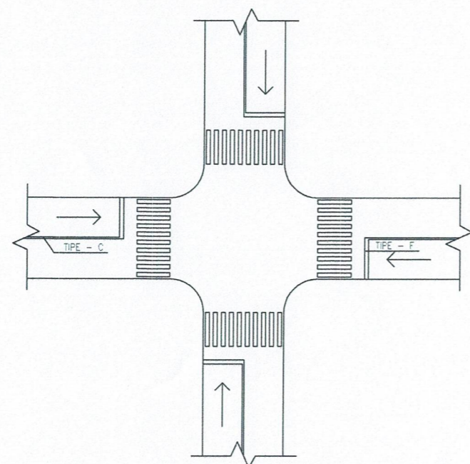
PERSIMPANGAN UNTUK PEJALAN KAKI
