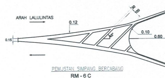
PENGGABUNGAN SIMPANG BER CABANG RM - 6 B
