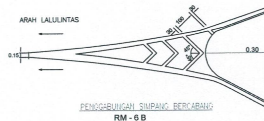
PERSIMPANGAN BER CABANG RM - 6 A
